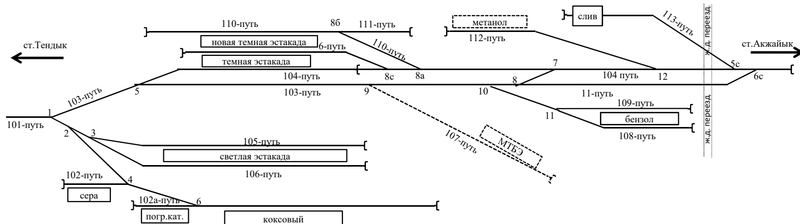
Схема подъездного пути ТОО "АНПЗ" на территории завода на 1 квартал 2020 года
