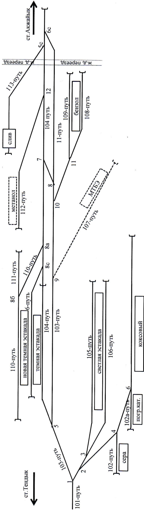
Схема подъездного пути ТОО "АНПЗ" на территории завода
